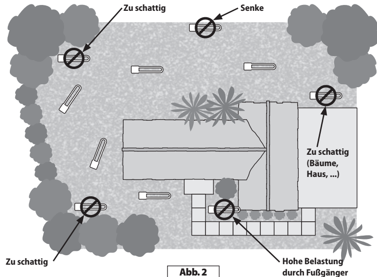
Abb. 2 Auswahl des Sensor-Standortes
